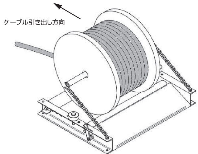
DR-6型(飛出し防止金具取付け例)
